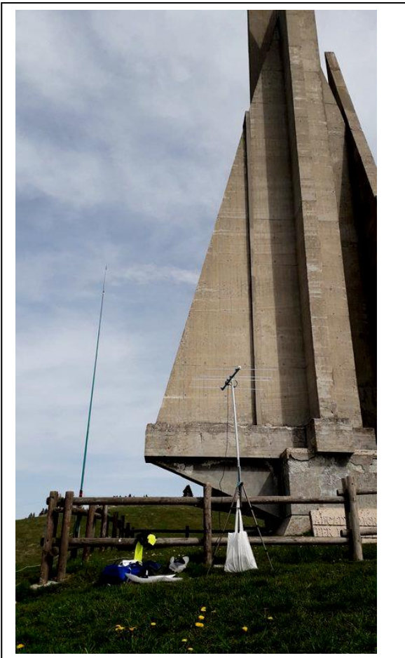
La verticale e la yagi posizionate sotto il monumento. La yagi punta a sud.
